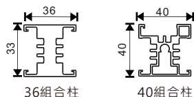
36組合柱
